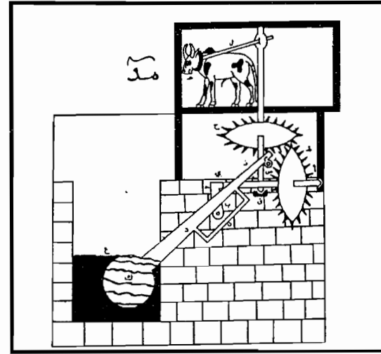
الجزاری کی بنائی ہوئی چوتھی واٹر ریزنگ مشین
