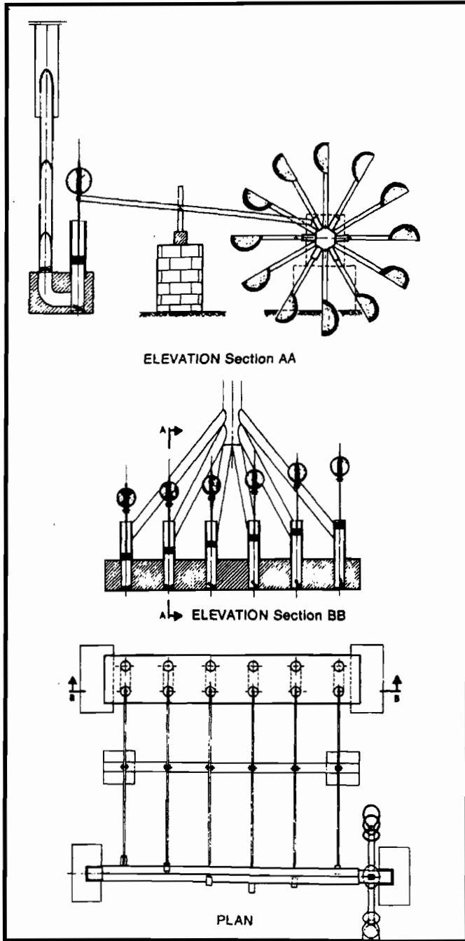
تقی الدین کا بیان کیا ہوا پانی سے چلنے والا چھ سلنڈر والا اسٹین پمپ (سولہویں صدی)
